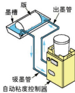
①直接循環控制方式
