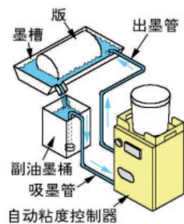
②採用副油墨桶進行溢流式循環控制方式
