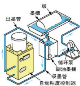
③用循環泵通過副油墨桶進行溢流式循環控制方式
